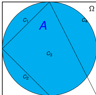
Figura 2: Ilustração – Teorema de probabilidade total.
