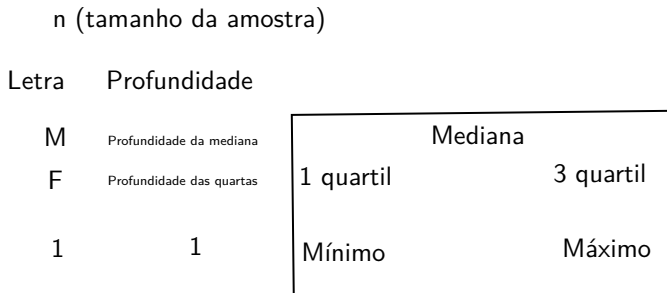
Figura 4: Diagrama de resumo de cinco números.
