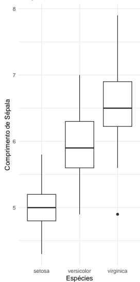
Diagrama de caixa
